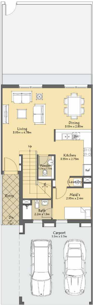
GROUND LEVEL الطابق الأرضي
