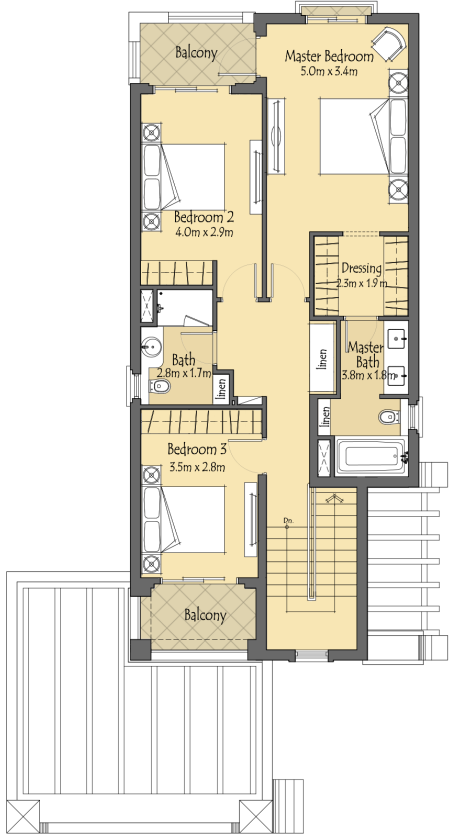
FIRST LEVEL الطابق الأول
