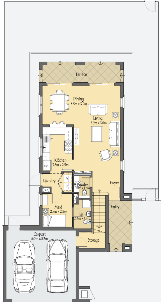
GROUND LEVEL الطابق الأرضي
